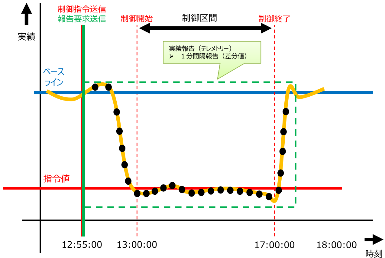
【制御指令と報告要求タイミングのイメージ】（二次調整力②相当）
