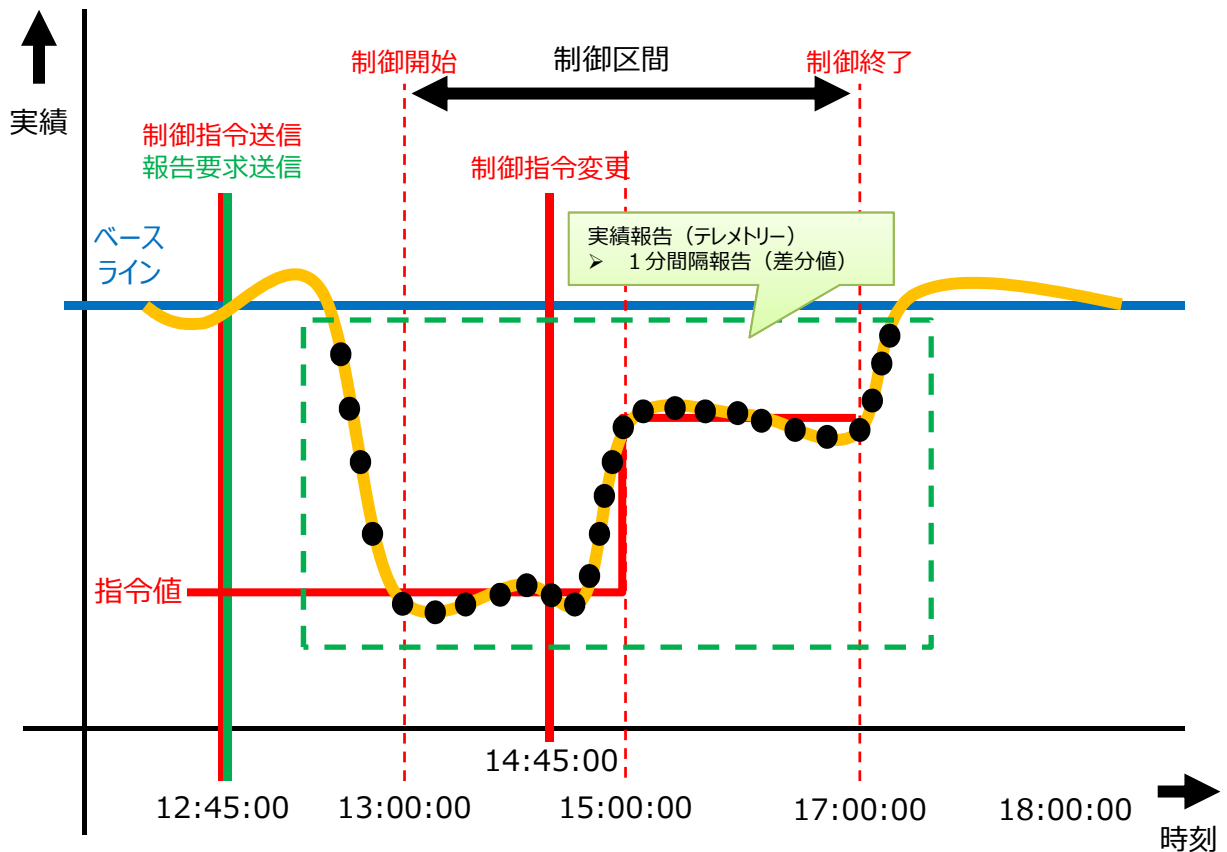
【制御指令変更と報告タイミングのイメージ】（三次調整力①相当）
