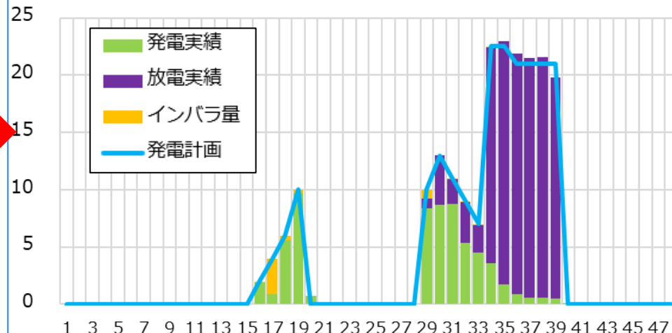
蓄電池制御（当日計画変更後）
