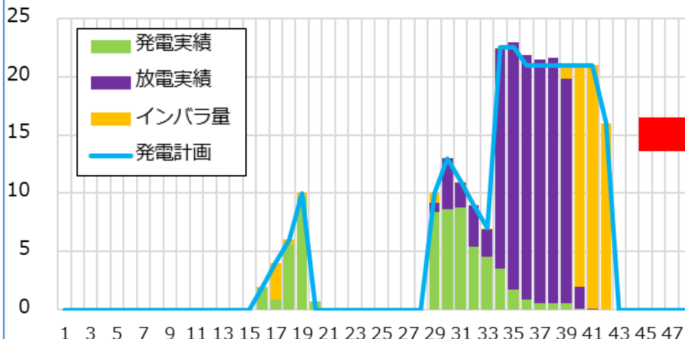
蓄電池制御（当日計画変更前）
