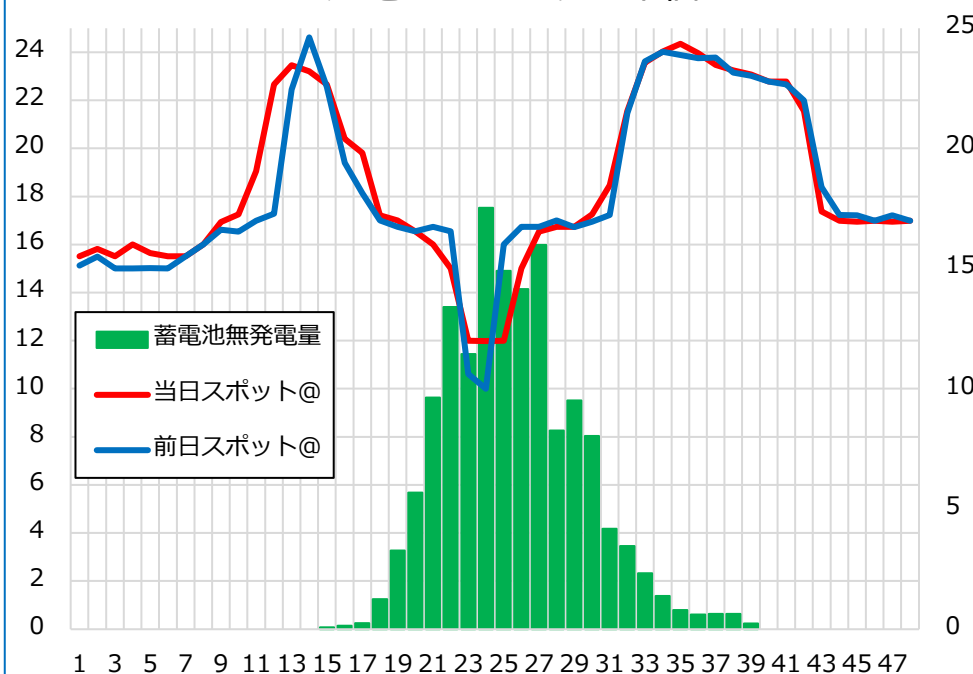
発電量 & スポット単価
