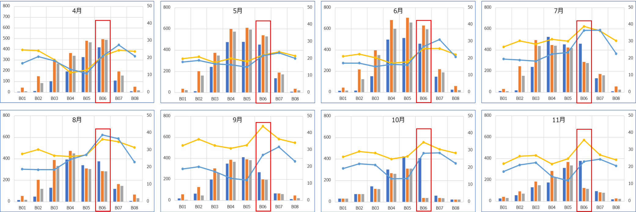
■ 募集量 ■ 入札量 ■ 約定量 — ΔkW+V1 — JEPX単価
