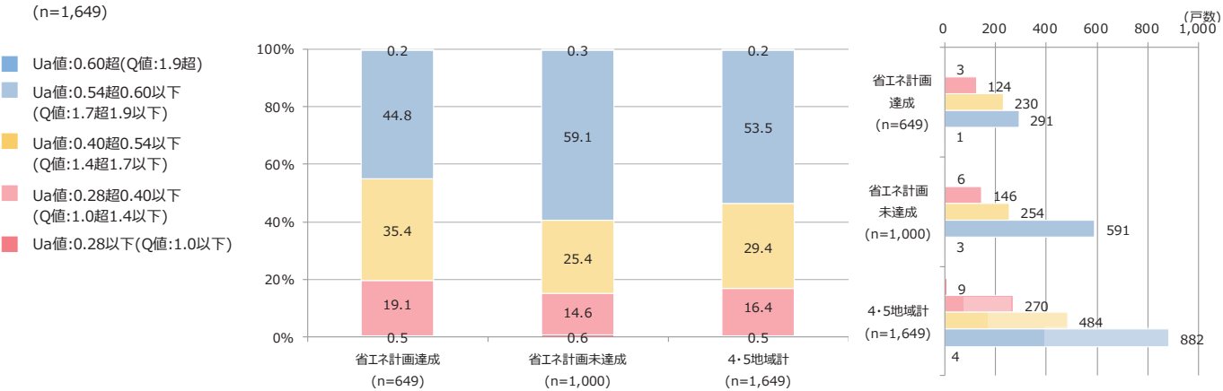
外皮性能の分布と構成比（4・5地域）
