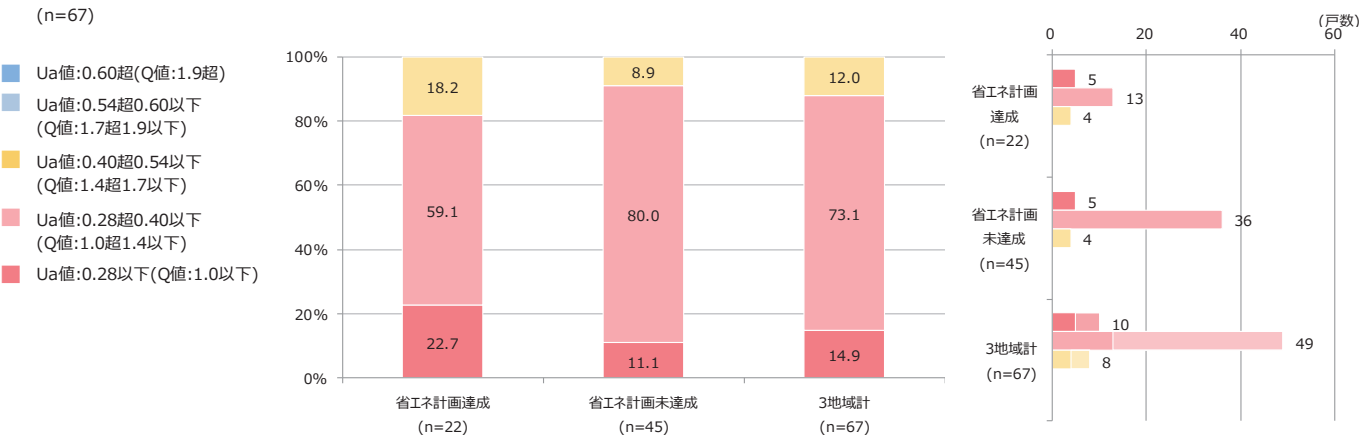
外皮性能の分布と構成比（3地域）
