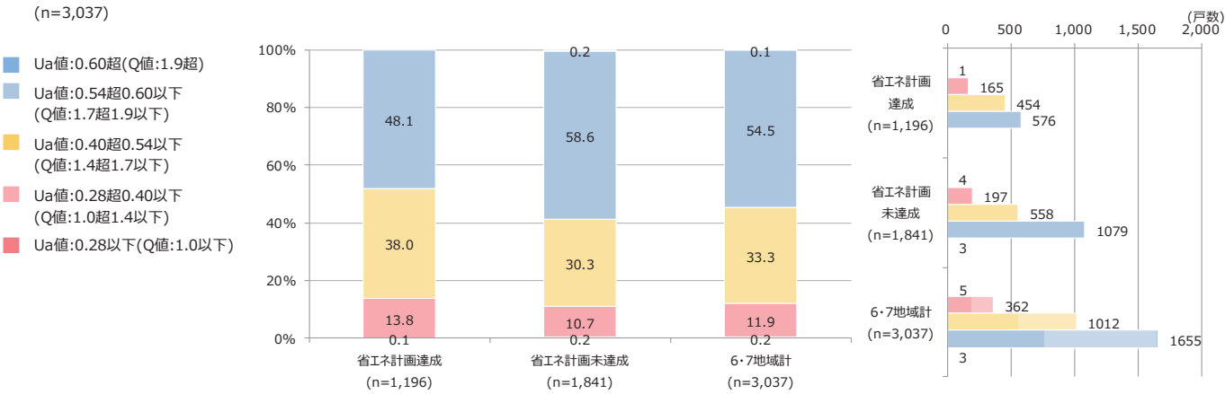
外皮性能の分布と構成比（6・7地域）
