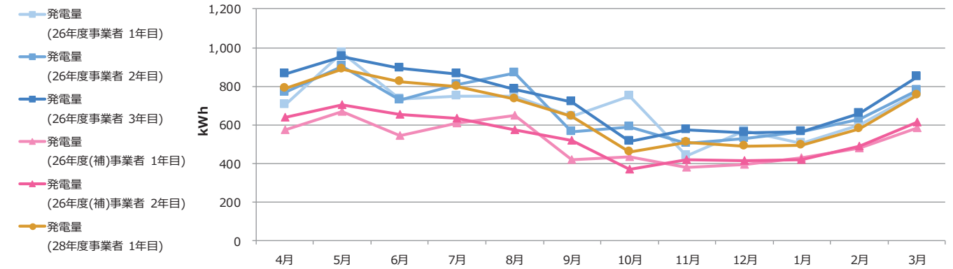
発電量の推移
