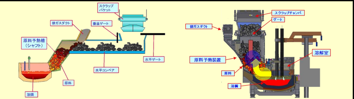
図 1 ECOARCTM、ECOARC-light概念図
